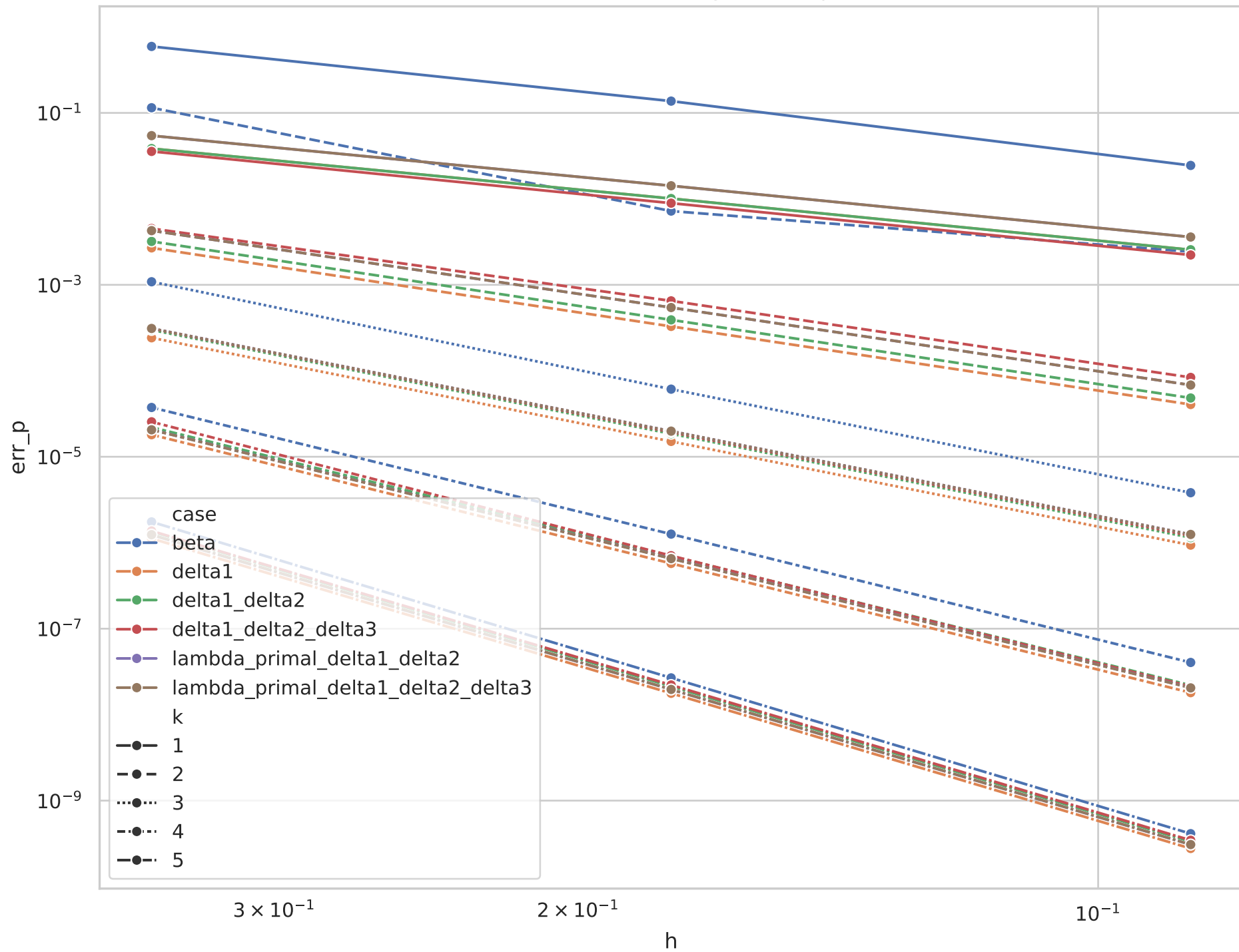
Lista 3 2D - convergência de p
